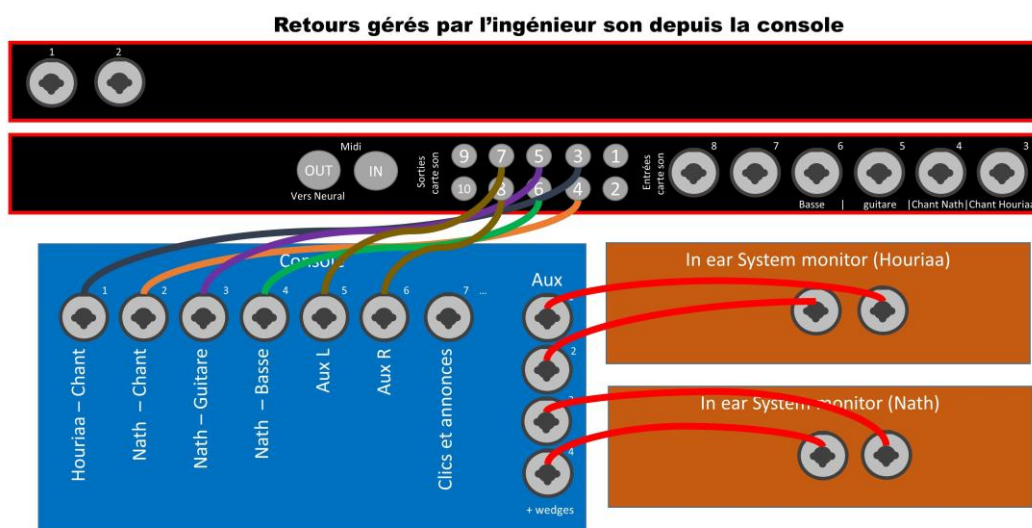
Figure 2 - Illustration patch (retours in ears gérés par l'ingénieur son depuis la console)
