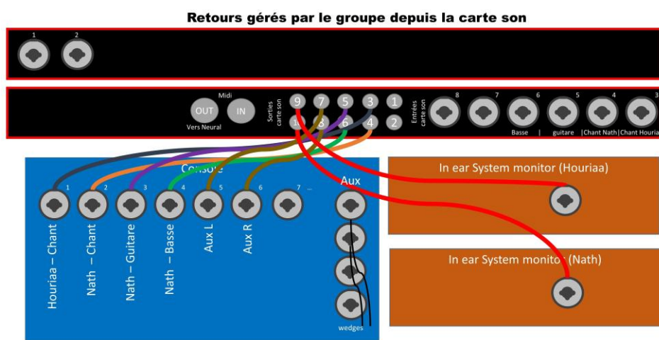
Figure 1 - Illustration patch (retours in ears gérés par le groupe depuis la carte son)
